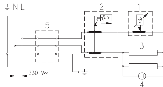
Diagrama eléctrico
