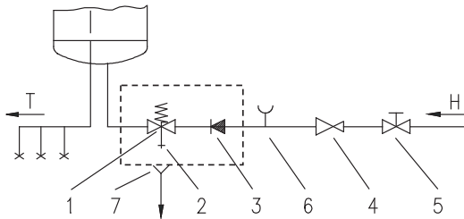
Sistema abierto (libre de presión)
