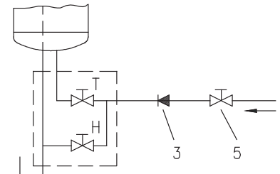
Sistema cerrado (a presión)
